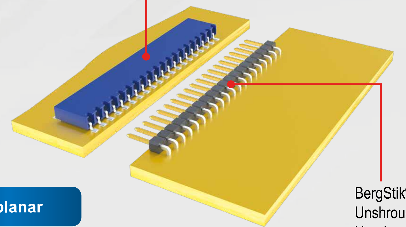
Dubox® Receptacle
